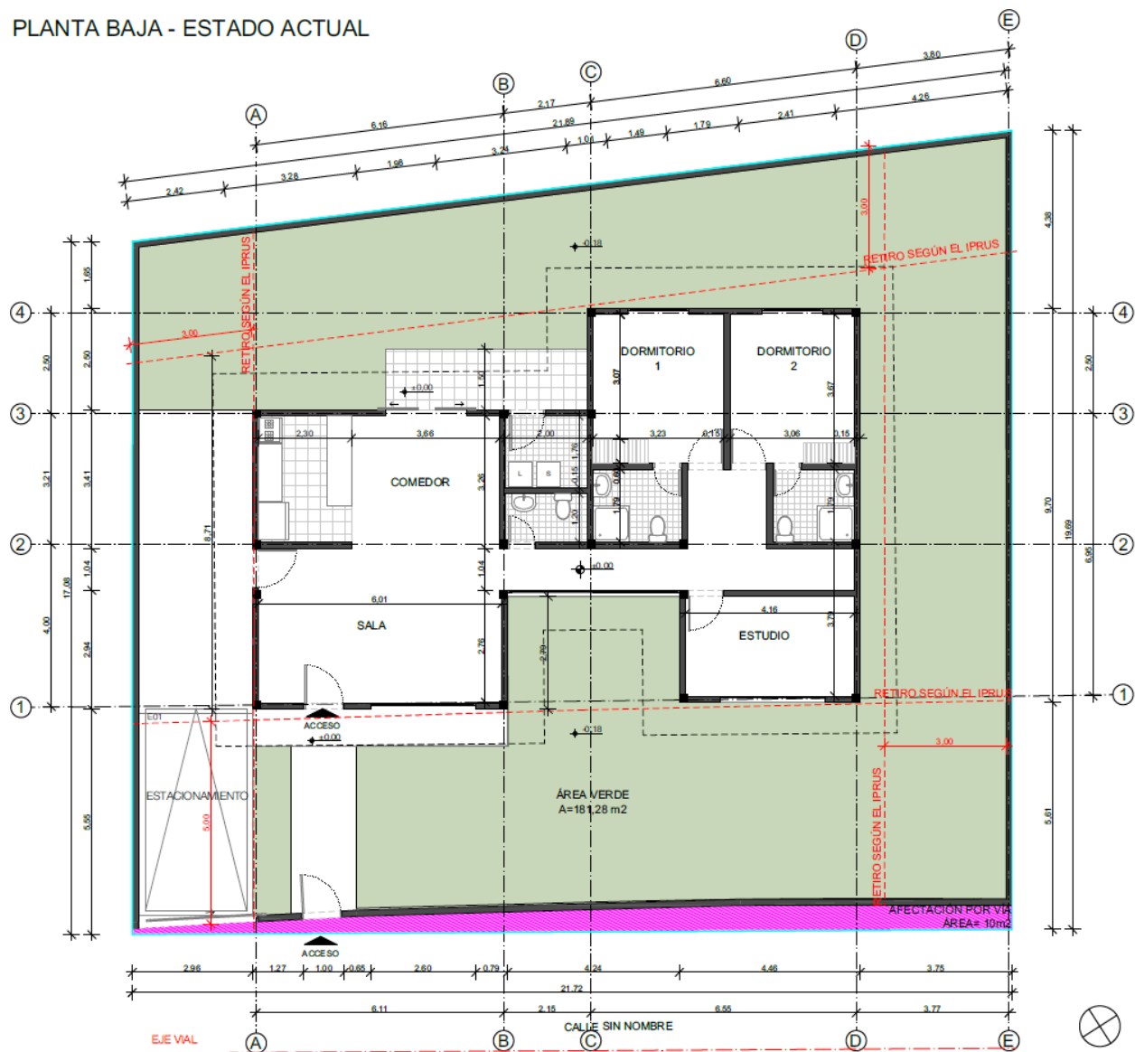
Planta baja-estado actual
