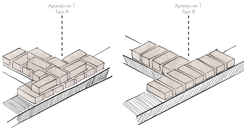
Fig. 2.2.16 | Unión entre tabiques de adobe. | Fuente: Autoría Propia. (2024).
