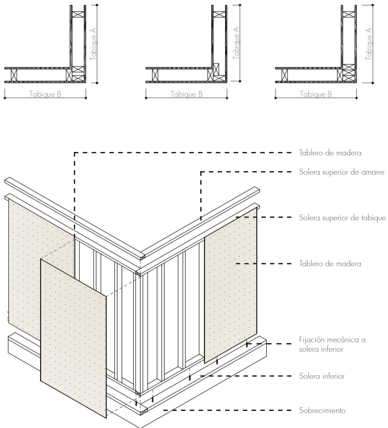
Fig. 3.3.10 | Diferentes tipos de uniones entre tabiques con bastidores A. | Fuente: Autoría Propia (2024).
