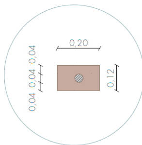
BLOQUE Material: Tierra Comprimida
