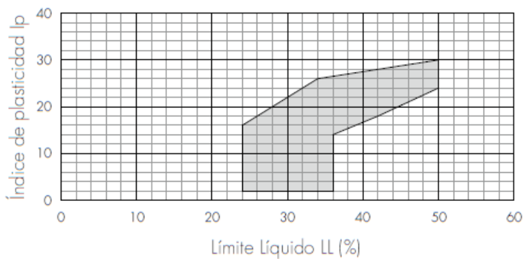
Fig. 3.2.14 | Zona recomendada en el diagrama de plasticidad de tierras para fabricación de BTC. | Fuente: Minke, (2006)
