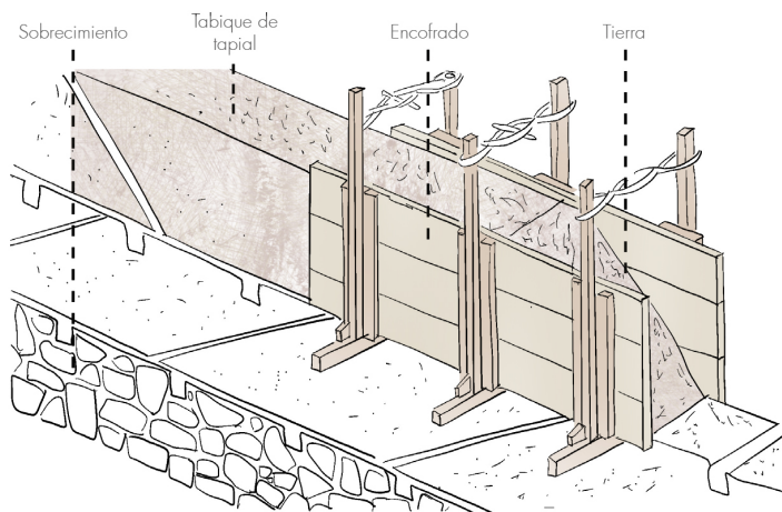
Fig. 2.4.10 | Encofrado deslizante horizontal. | Fuente: Autoría Propia (2024).
