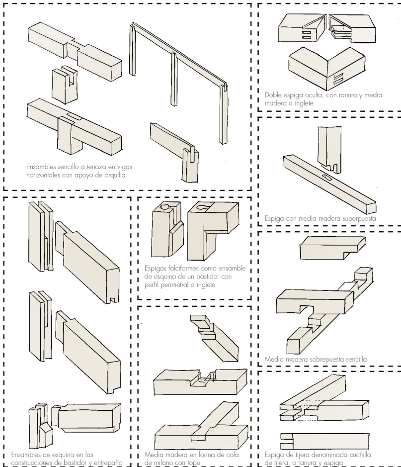
Fig. 3.3.19 | Ejemplos de ensamblajes en ángulo y en cruz - A. | Fuente: Autoría Propia (2024).
