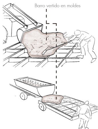
Fig. 2.2.11 | Fabricación de adobes con moldes múltiples. | Fuente: Autoría Propia. (2024).
