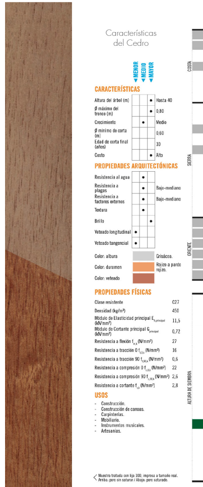
Fig.3.3.22 | Características del cedro. | Fuente: Arpi, et al. (2018).
