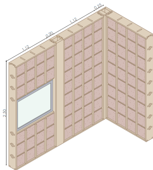
Unión entre tabiques en encuentro en esquina y tabique con ventana
