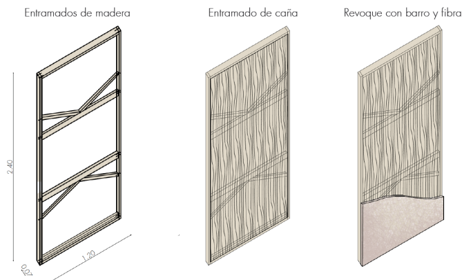
Fig. 2.5.20 | Quinchá prefabricada - Instituto Nacional de Investigación y Normalización de la Vivienda - ININVI. Fuente: Autoría Propia (2024).
