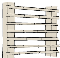
d) Entramado horizontal separado sobre estructura.
