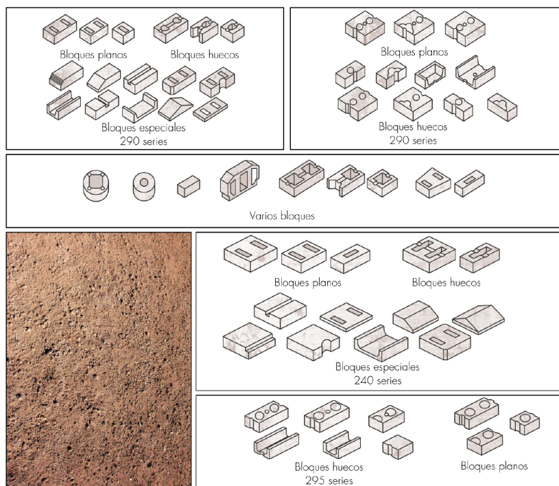
Fig. 3.2.10 | Ejemplos de diferentes tipos de bloques de tierra comprimida articulados y bloques accesorio. Fuente: Autoría Propia (2024).
