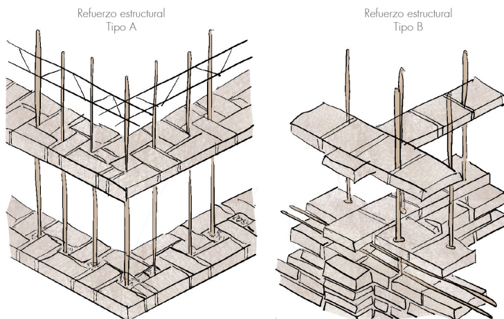
Fig. 2.2.18 | Refuerzo de tabiques de adobe con estructuras auxiliares. | Fuente: Autoría Propia. (2024).
