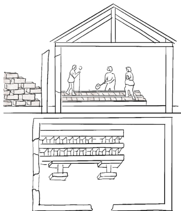
Fig. 3.2.5 | Francois Cointeraux - Bloques de tierra comprimida, 1803. | Fuente: Autoría Propia (2024).
