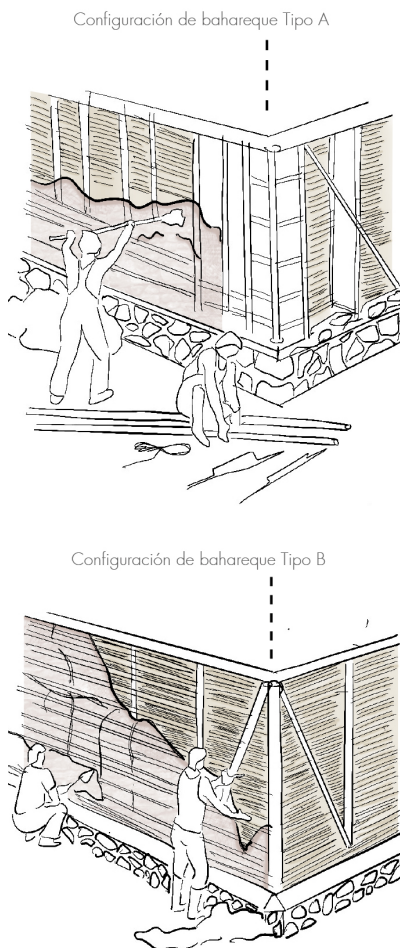
Fig. 2.3.6 | Ejemplos de entramados en tabiques de bahareque. | Fuente: Autoría Propia. (2024).
