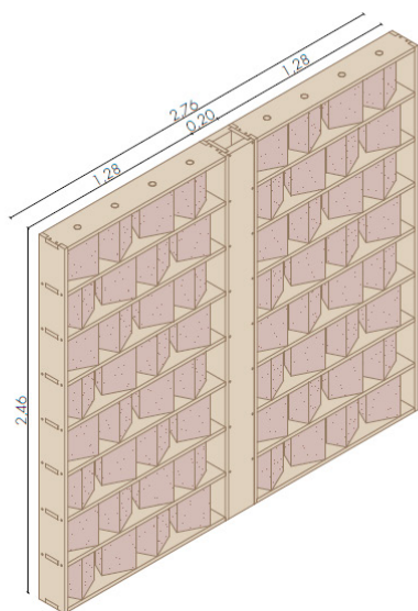
Unión entre Tabiques
