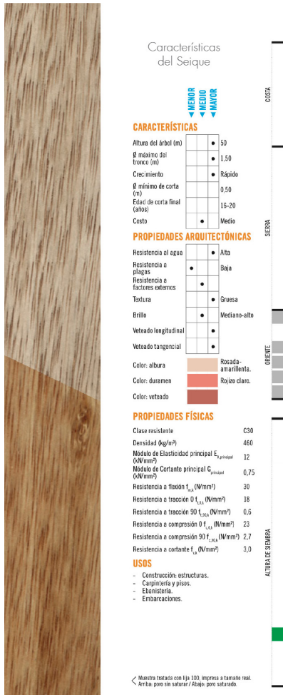
Fig.3.3.21 | Características del seique. | Fuente: Arpi, et al. (2018).
