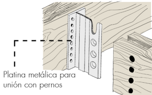
Fig.3.3.12 | Unión con ángulos. | Fuente: Autoría Propia (2024).
