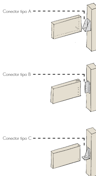
Fig.3.3.13 | Unión con conectores. | Fuente: Autoría Propia (2024).
