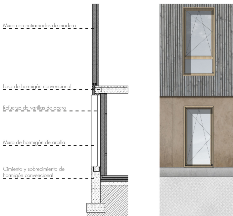
Fig. 2.5.18 | Detalle de tabique de hormigón de arcilla construido en 2028 para el proyecto Pépinière d'entreprises à Saint-Clair-de-la-Tour, Isère, Reach & Scha. | Fuente: Autoría Propia (2024).
