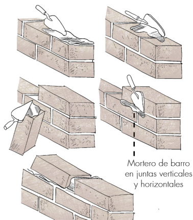
Fig. 2.2.15 | El trabajo con el mortero es importante en la configuración de tabiques de adobe. | Fuente: Autoría Propia. (2024).
