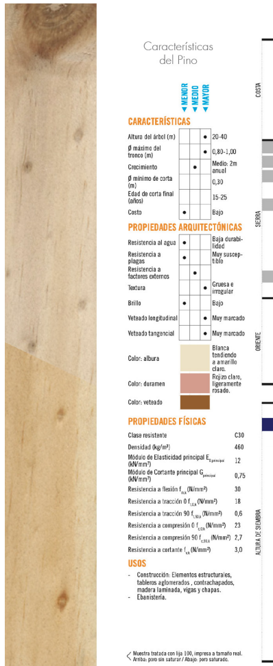
Fig.3.3.27 | Características del pino. Fuente: Arpi, et al. (2018).
