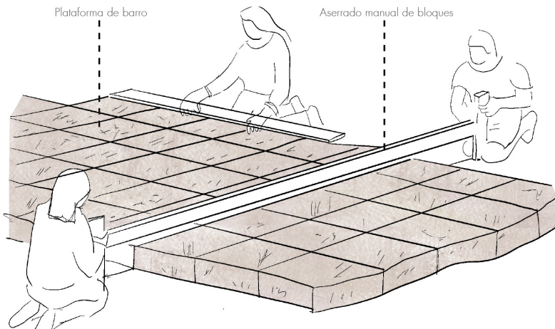
Fig. 2.2.12 | Fabricación de adobes aserrados. | Fuente: Autoría Propia. (2024).
