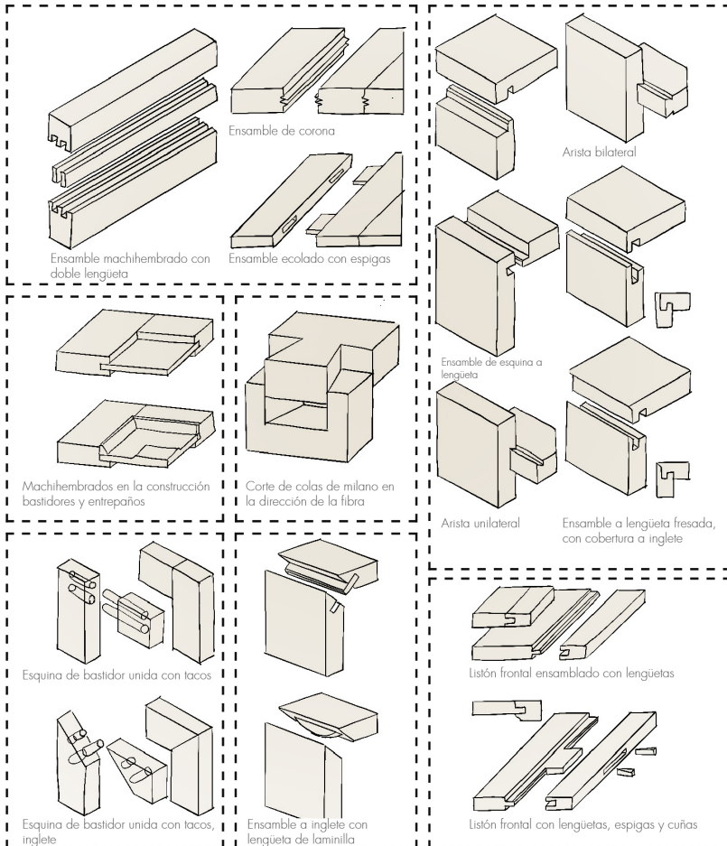
Fig. 3.3.20 | Ejemplos de ensamblajes planos. | Fuente: Autoría Propia (2024).
