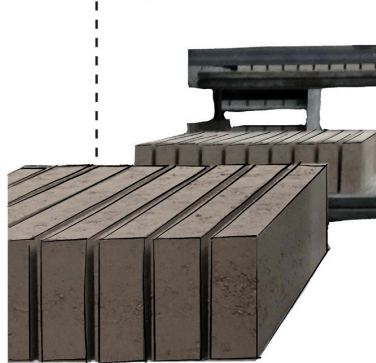
Fig. 2.5.14 | Tapialblock, bloque de tierra compactada de 8 x 100 x 15 cm. | Fuente: Autoría Propia (2024). A partir de: www.fetdeterra.com
