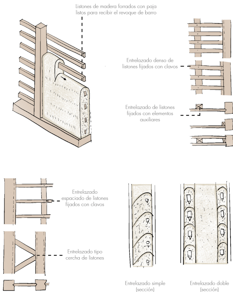
Fig. 2.3.14 | Ejemplos de diferentes técnicas de colocación del barro con la paja sobre el entramado. Fuente: Autoría Propia (2024).
