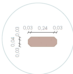
BLOQUE TIPO 2 Material: Tierra Comprimida Cantidad: 32 unidades
