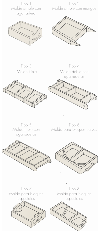
Fig. 2.2.5 | Diferentes moldes para adobes tradicionales. | Fuente: Autoría Propia. (2024).
