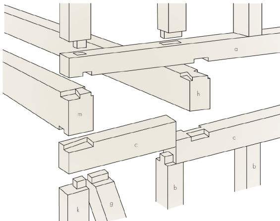
Fig. 3.3.16 | Unión con ensambles. | Fuente: Autoría Propia (2024).
