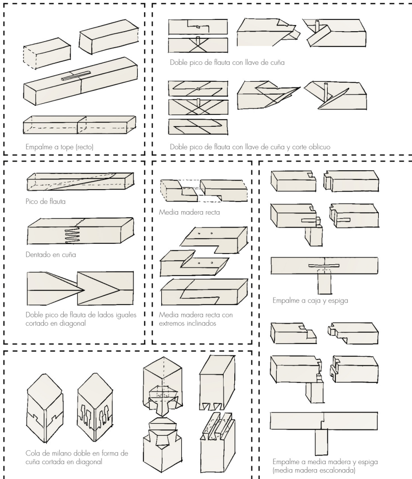
Fig. 3.3.17 | Ejemplos de ensamblajes longitudinales - B. | Fuente: Autoría Propia (2024).
