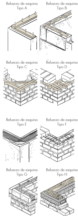
Fig. 2.2.19 | Refuerzo de tabiques de adobe con estructuras auxiliares. | Fuente: Autoría Propia. (2024).
