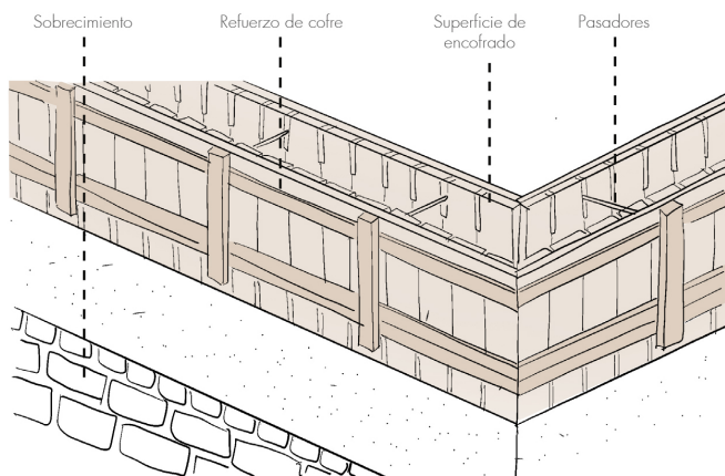
Fig. 2.4.12 | Encofrado integral horizontal. | Fuente: Autoría Propia (2024).
