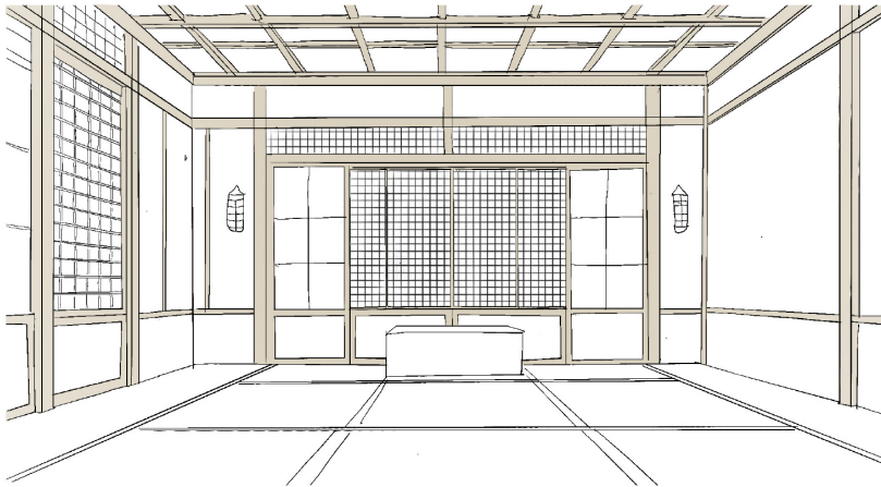
Fig. 3.3.4 | Tabiques tradicionales en la arquitectura japonesa modulados a partir de las dimensiones del Tatami. | Fuente: Autoría Propia (2024).
