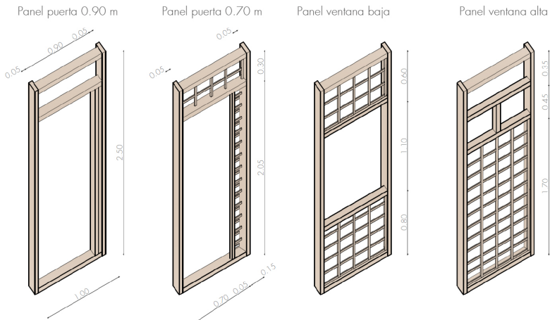
Fig. 2.5.23 | Tipos de paneles. | Fuente: Autoría Propia (2024).
