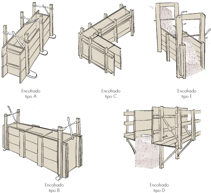
Fig. 2.4.9 | Ejemplos de diferentes sistemas de encofrados. | Fuente: Autoría Propia (2024).
