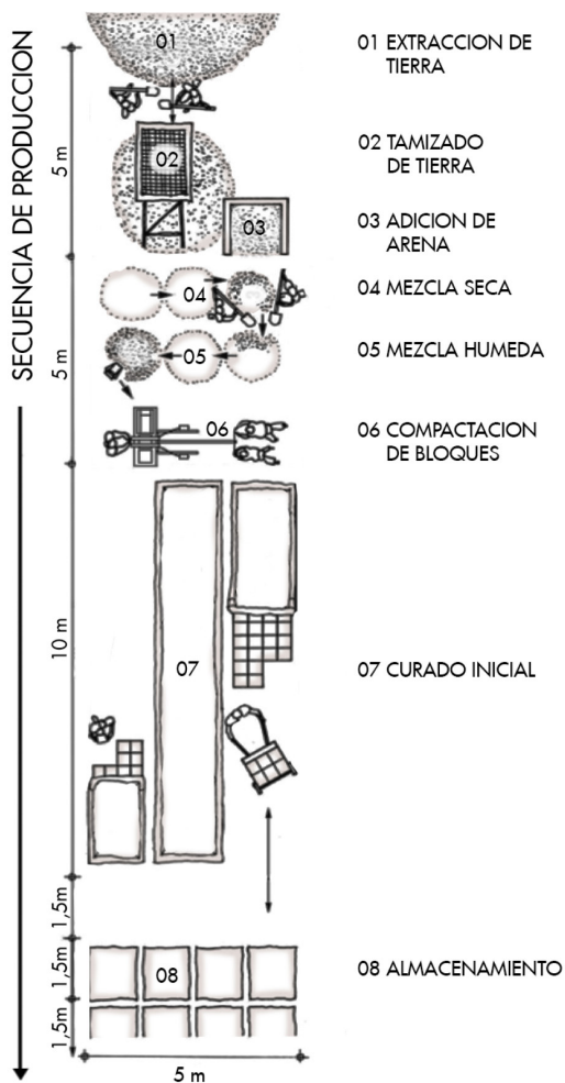
Fig.3.2.3 | Cadena de proceso de elaboración de BTC mediante una prensa manual. | Fuente: Autoría Propia (2024).
