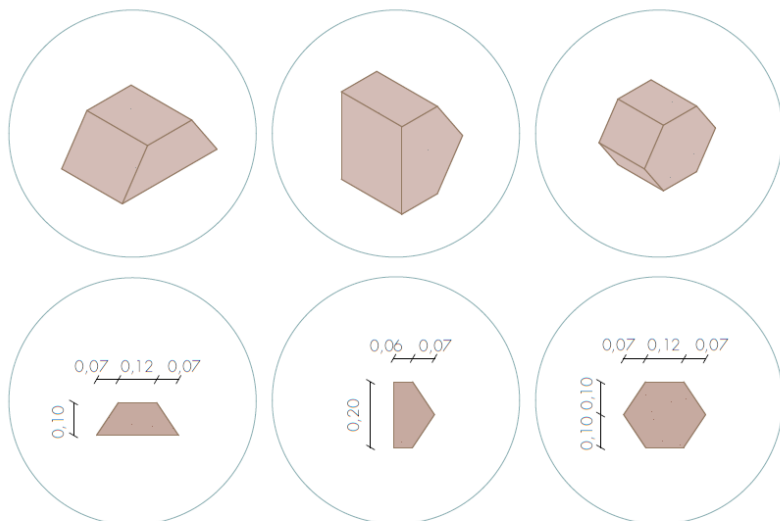
MITAD DE BLOQUE HEXAGONAL
