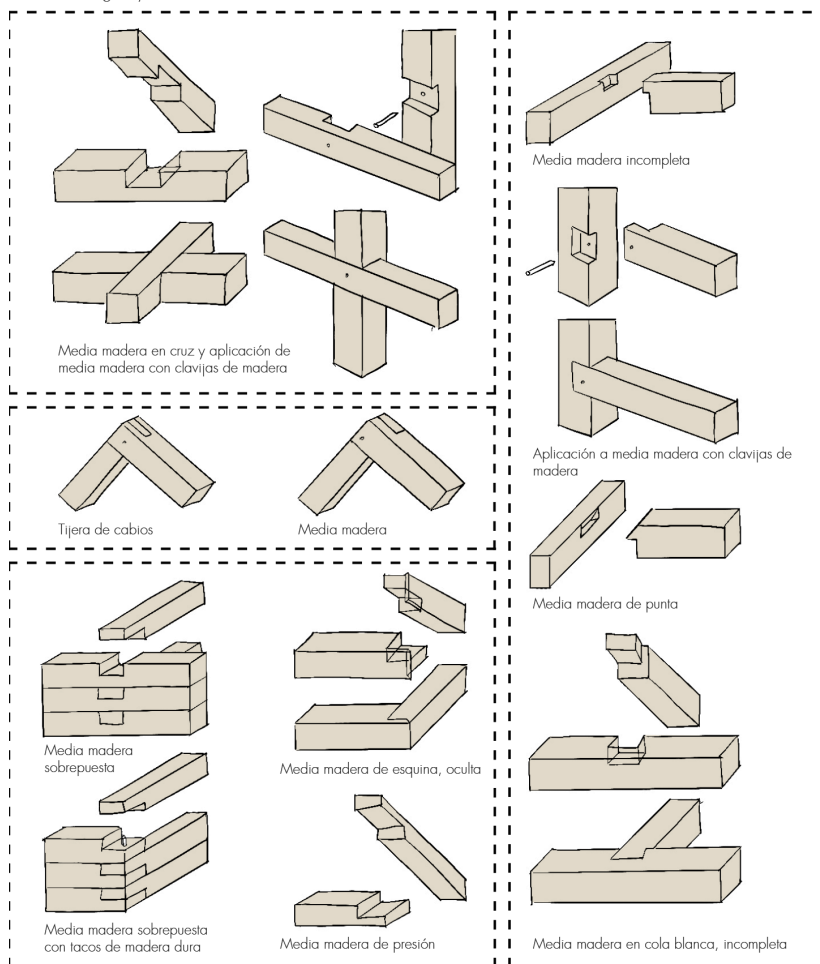
Fig. 3.3.19 | Ejemplos de ensamblés en ángulo y en cruz - B. | Fuente: Autoría Propia (2024).
