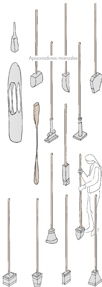
Fig. 2.4.17 | Apisonadores manuales. | Fuente: Autoría Propia (2024).
