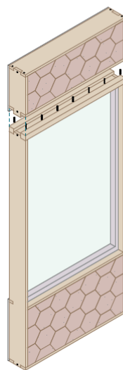
Paso 4 Instalación de tabique superior.
