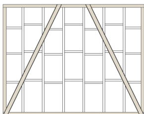
Rigidización con diagonales tipo C
