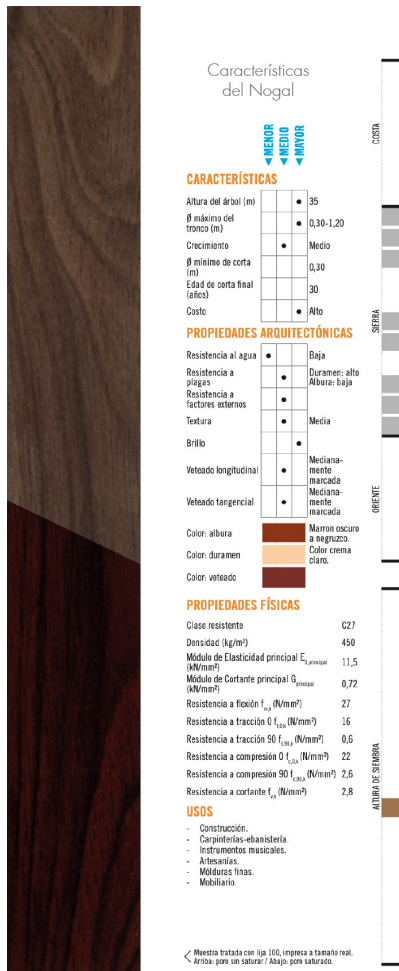
Fig.3.3.24 | Características del nogal. | Fuente: Arpi, et al. (2018).
