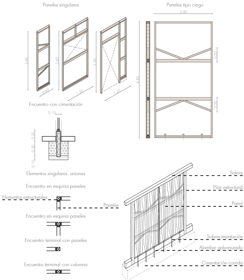
Fig. 2.5.21 | Detalles - Quincha prefabricada - Instituto Nacional de Investigación y Normalización de la Vivienda - ININVI. | Fuente: Autoría Propia (2024).
