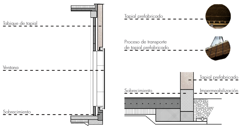
Fig. 2.5.12 | Es importante la Impermeabilización y el trabajo en sinergia con los elementos constructivos en hormigón armado. | Fuente: Autoría Propia (2024).
