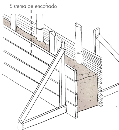
Fig. 2.4.1 | Ejemplo del proceso constructivo mediante encofrados de un tabique de tapial. | Fuente: Autoría Propia (2024).
