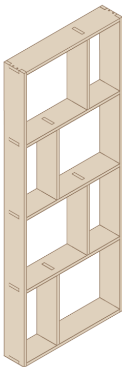
Armazón para muro de bloques
