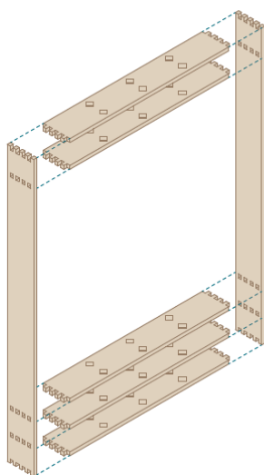
Paso 1 Tablones laterales e intermedios.
