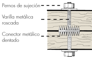
Fig.3.3.15 | Unión con conectores dentados. | Fuente: Autoría Propia (2024).
