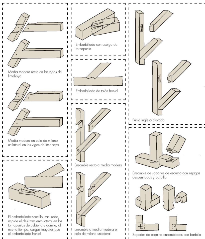
Fig. 3.3.18 | Ejemplos de ensamblajes oblicuos. | Fuente: Autoría Propia (2024).
