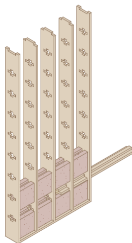
Paso 2 Sistema de trabado: tableros intermedios horizontales y bloques.
