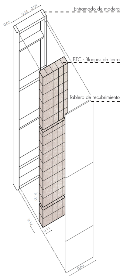
Fig. 2.5.7 | Tabi ques con BTC empleados por la oficina de arquitectura Schauer+Volhard en Alemania. | Fuente: Autoría Propia (2024).
