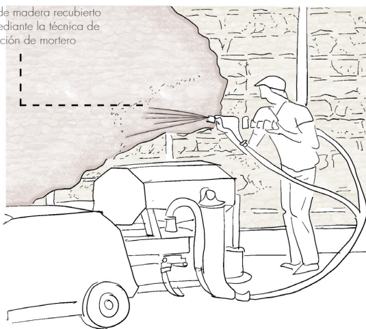
Fig. 2.3.4 | Técnica del mortero de barro proyectado sobre entramados. | Fuente: Autoría Propia. (2024).
