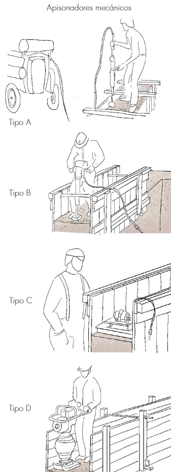
Fig. 2.4.18 | Apisonadores mecánicos. | Fuente: Autoría Propia (2024).
