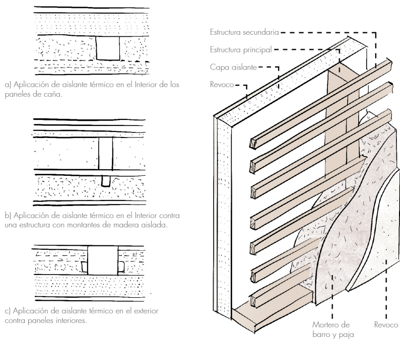
Fig. 2.3.8 | El comportamiento térmico de un tabique de bahareque puede ser optimizado en climas extremos. | Fuente: Autoría Propia. (2024).
