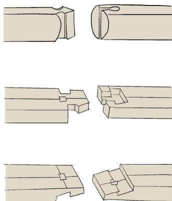
Fig. 3.3.3 | Ejemplos de ensamblajes del manual Ying-tsao Fashih. | Fuente: Autoría Propia (2024).
