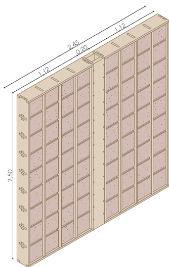
Unión entre Tabiques
