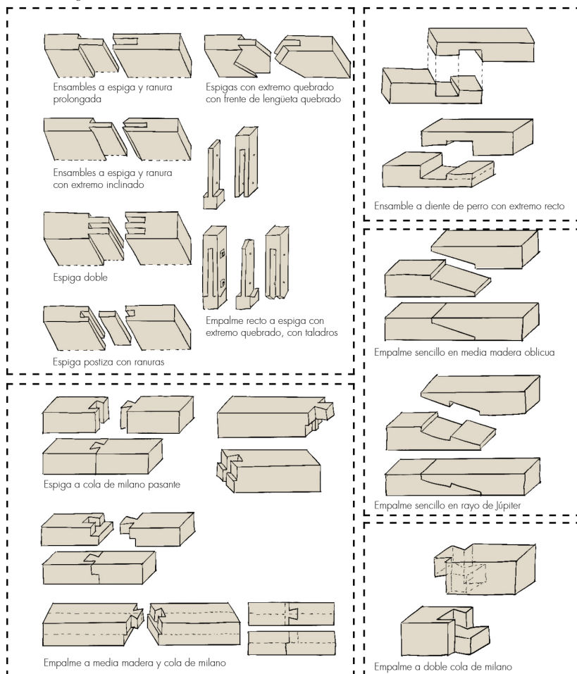
Fig. 3.3.17 | Ejemplos de ensamblajes longitudinales - A. | Fuente: Autoría Propia (2024).
