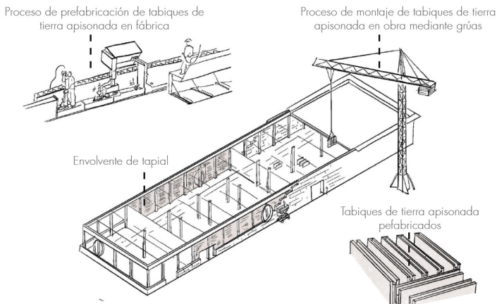
Fig. 2.5.11 | El uso de bloques prefabricados de tapial de gran formato en el proyecto Ricola Kräuterzentrum. | Fuente: Autoría Propia (2024).
