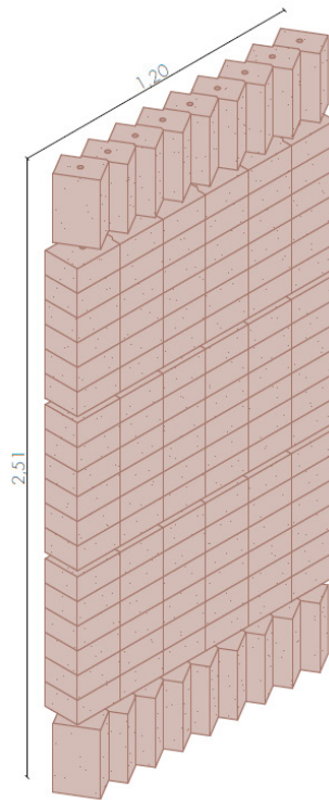
Muro de bloques
