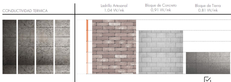
Fig. 3.2.18 | Comparación de las características sostenibles entre diferentes materiales convencionales y el BTC. Fuente: Autoría Propia (2024).
