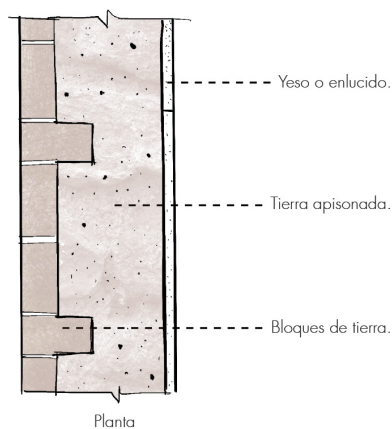
Fig. 2.4.3 | Ejemplo de muro de tapial y de bloques de tierra. | Fuente: Autoría Propia (2024).
