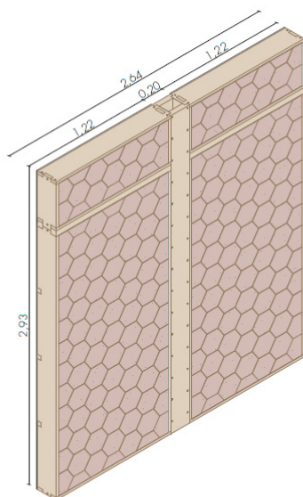
Unión entre Tabiques
