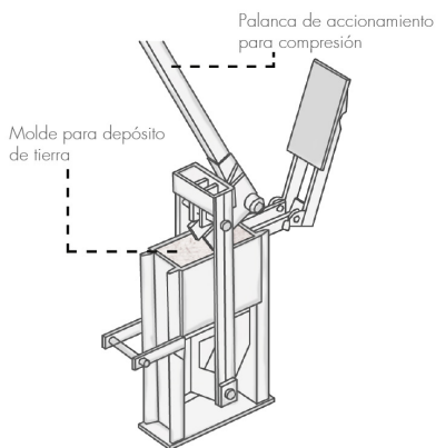
Fig. 3.2.6 | Prensa de bloques de tierra comprimida CINVA RAM. | Fuente: Autoría Propia (2024).
