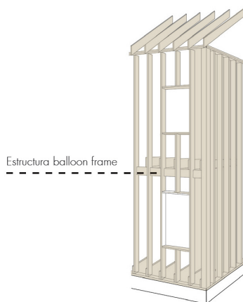
Fig.3.3.5 | Sistema Balloon frame. | Fuente: Autoría Propia (2024).
