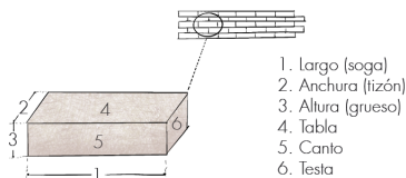
Fig.3.2.9 | Nomenclatura habitualmente utilizada para designar las partes de los BTC según la norma UNE 41410:2023. | Fuente: Autoría Propia (2024).
