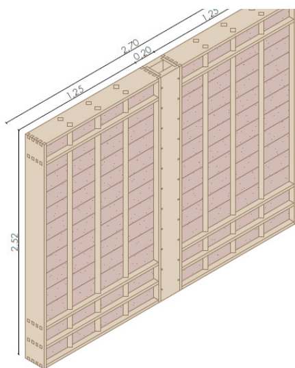
Unión entre Tabiques
