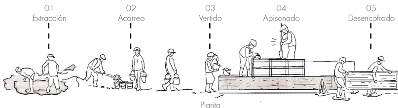
Fig. 2.4.2 | Construcción de tabiques con tapial. | Fuente: Autoría Propia (2024).
