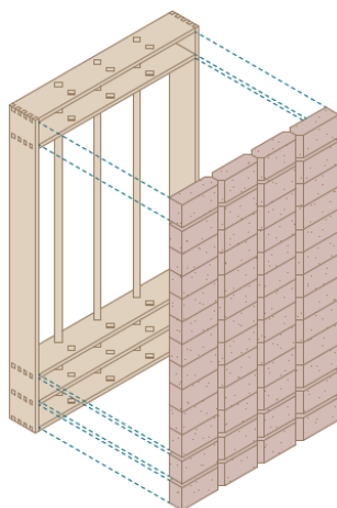
Paso 3 Sistema de trabado: tablones intermedios, listones posteriores y bloques.
