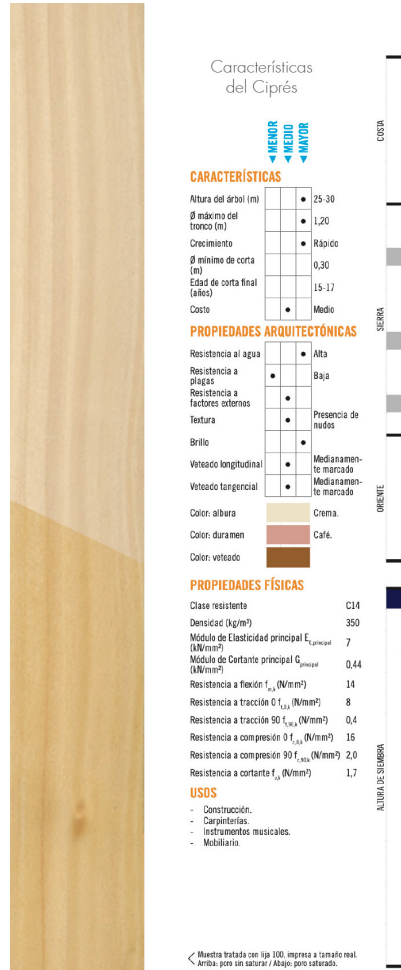
Fig.3.3.28 | Características del ciprés. Fuente: Arpi, et al. (2018).
