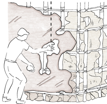
Entramado de caña recubierto de barro mediante la técnica de COB
