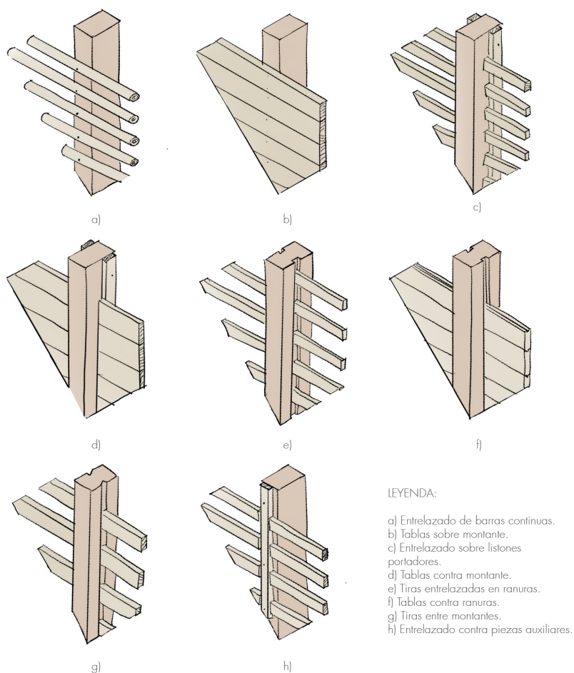
Fig. 2.3.10 | Configuración de la estructura con diferentes materiales y uniones. | Fuente: Autoría Propia. (2024).
