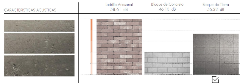
Fig. 3.2.17 | Comparación del comportamiento acústico entre diferentes materiales convencionales y el BTC. | Fuente: Autoría Propia (2024).
