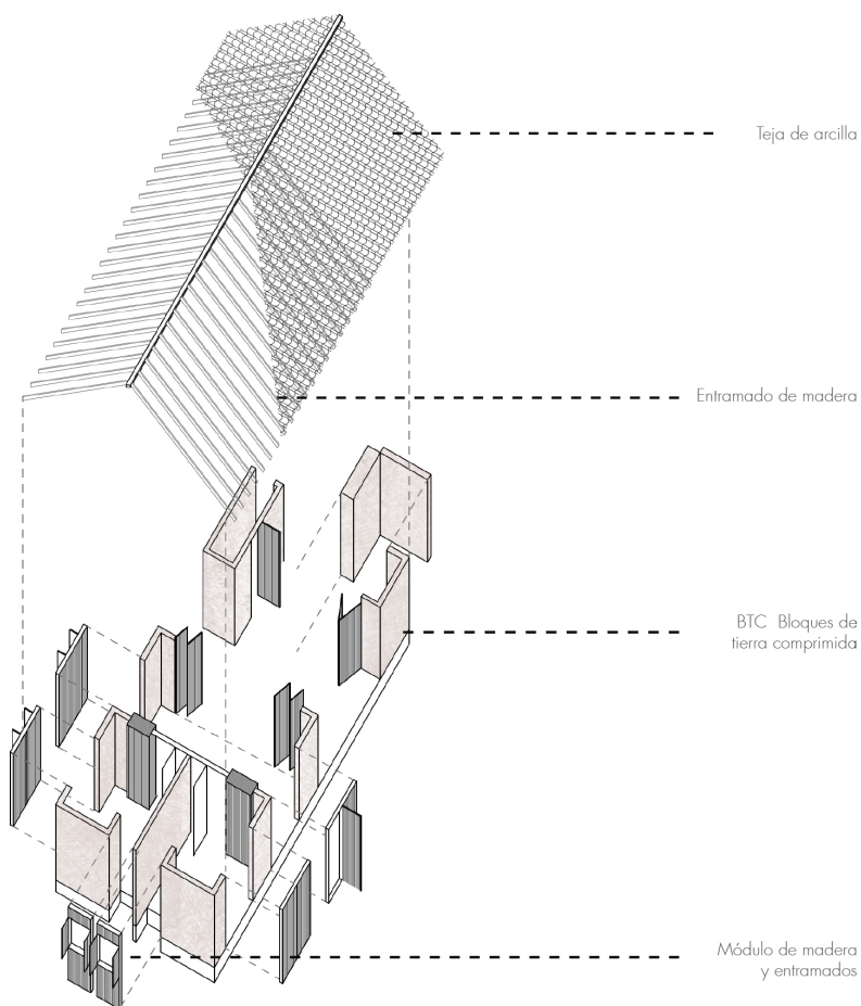
Fig. 2.5.3 | BTC, Axonometría de proyecto Kirinda Houses. | Fuente: Autoría Propia (2024).
