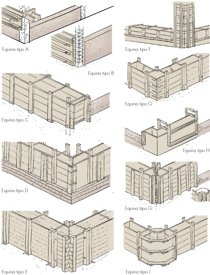
Fig. 2.4.16 | Los encofrados y el tratamiento de las esquinas. | Fuente: Autoría Propia (2024).
