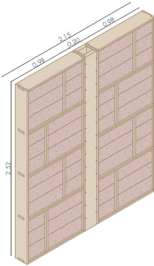
Unión entre Tabiques
