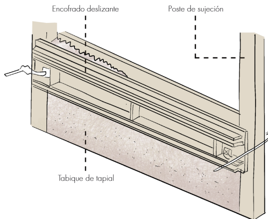
Fig. 2.4.11 | Encofrado deslizable vertical. | Fuente: Autoría Propia (2024).
