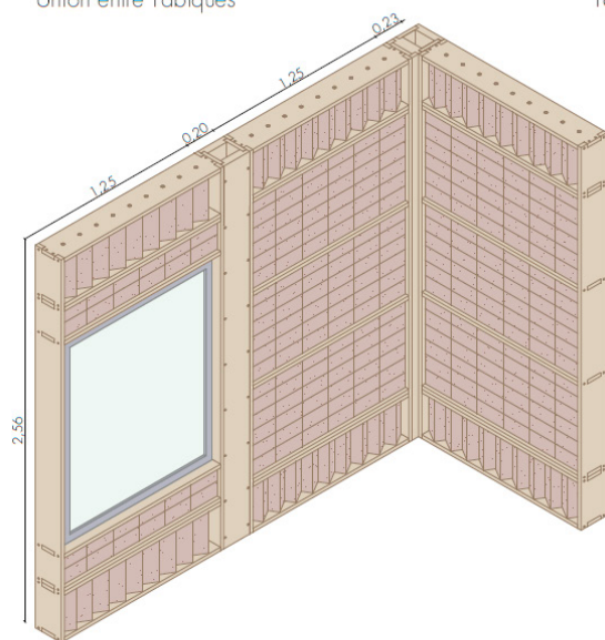
Unión entre tabiques en encuentro en esquina y tabique con ventana
