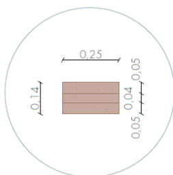
BLOQUE TIPO 1 Material: Tierra Comprimida Cantidad: 28 unidades
