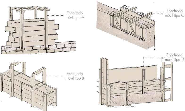
Fig. 2.4.14 | Diferentes tipos de encofrados móviles. | Fuente: Autoría Propia (2024).
