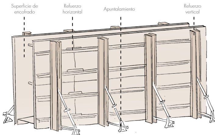
Fig. 2.4.13 | Encofrado integral vertical. | Fuente: Autoría Propia (2024).
