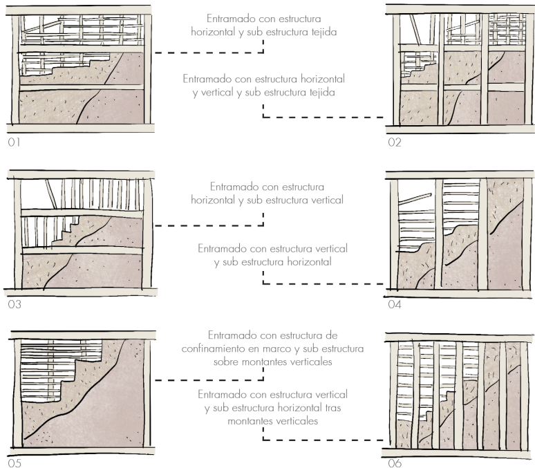
Fig. 2.3.7 | Variantes de la técnica del bahareque. | Fuente: Autoría Propia. (2024).
