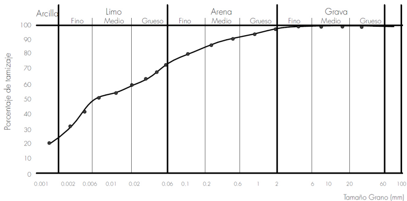
Fig. 2.2.3 | Curva granulométrica optimizada para adobes. | Fuente: Gernot M. (2006).
