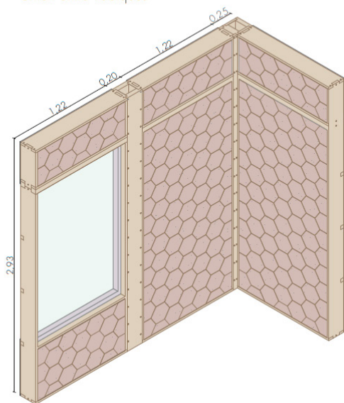
Unión entre tabiques en encuentro en esquina y tabique con ventana
