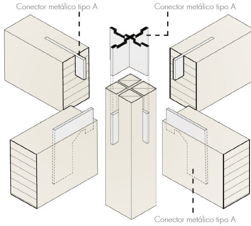
Fig. 3.3.14 | Unión con conectores múltiples. | Fuente: Autoría Propia (2024).
