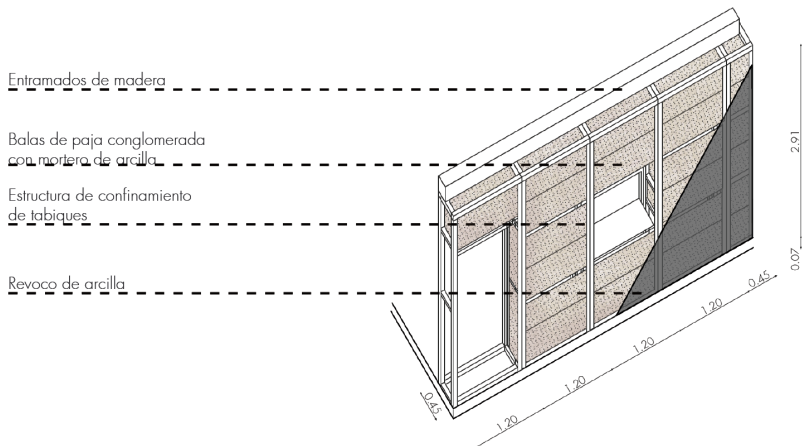
Fig. 2.5.9 | Tabi ques con elementos compuestos con paja y revocos de arcilla. | Fuente: Autoría Propia (2024).
