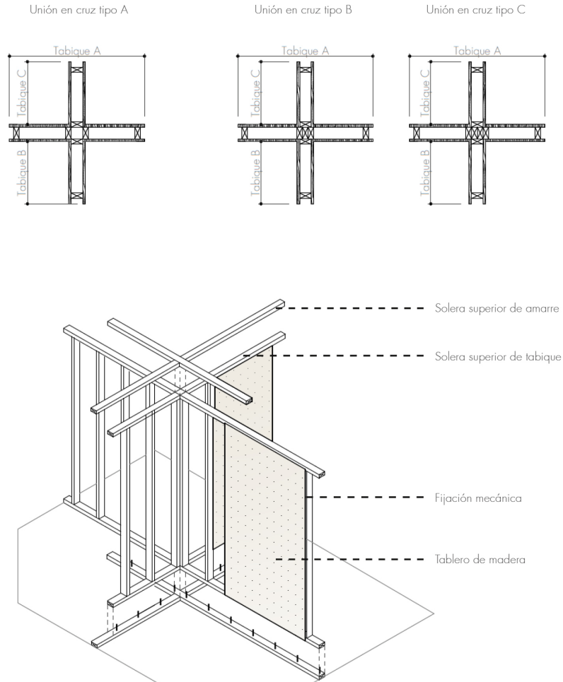
Fig. 3.3.10 | Diferentes tipos de uniones entre tabiques con bastidores C. | Fuente: Autoría Propia (2024).
