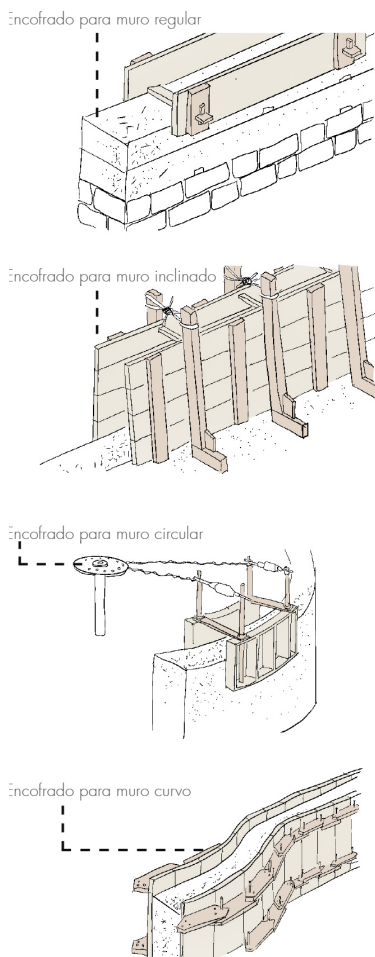
Fig. 2.4.15 | Encofrados con diferentes respuestas formales. | Fuente: Autoría Propia (2024).
