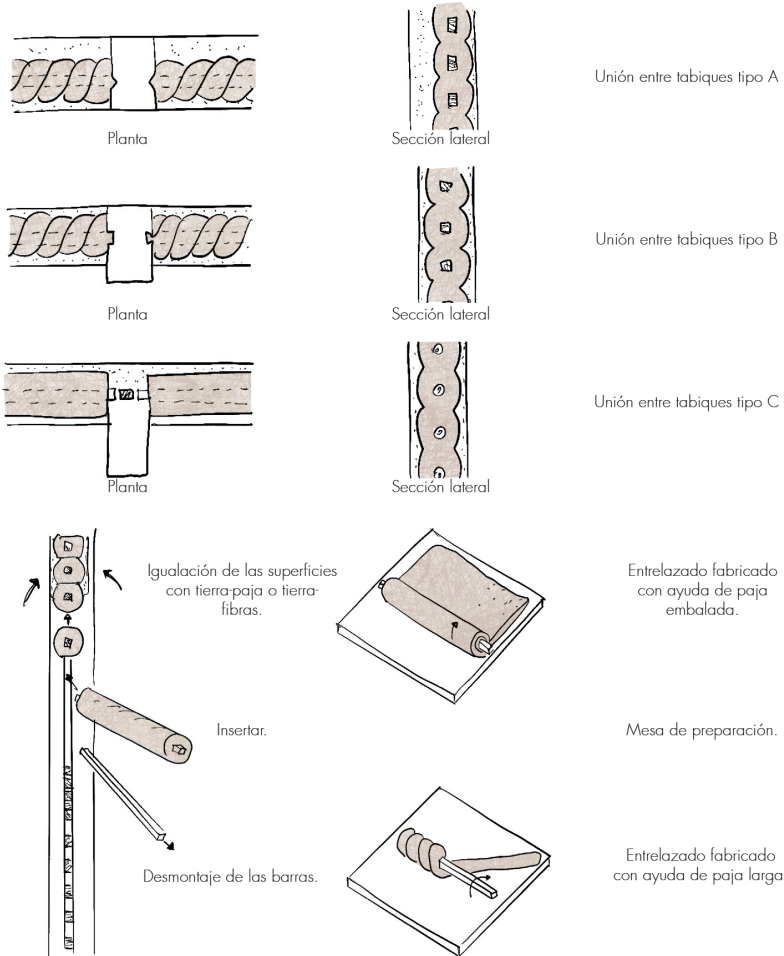
Fig. 2.3.14 | Ejemplos de diferentes técnicas de colocación del barro con la paja sobre el entramado. Fuente: Autoría Propia (2024).
