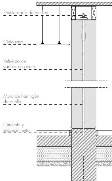
Fig. 2.5.17 | Detalle de tabique de hormigón de arcilla construido en 2018 para el proyecto Groupe scolaire Paul-Bayrou à Saint-Antonin-Noble-Val, Tarnet. | Fuente: Autoría Propia (2024).
