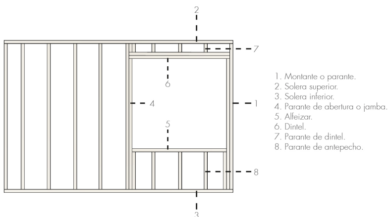
Fig. 3.3.8 | Tabique de entramado vertical con bastidores de madera. | Fuente: Autoría Propia (2024).
