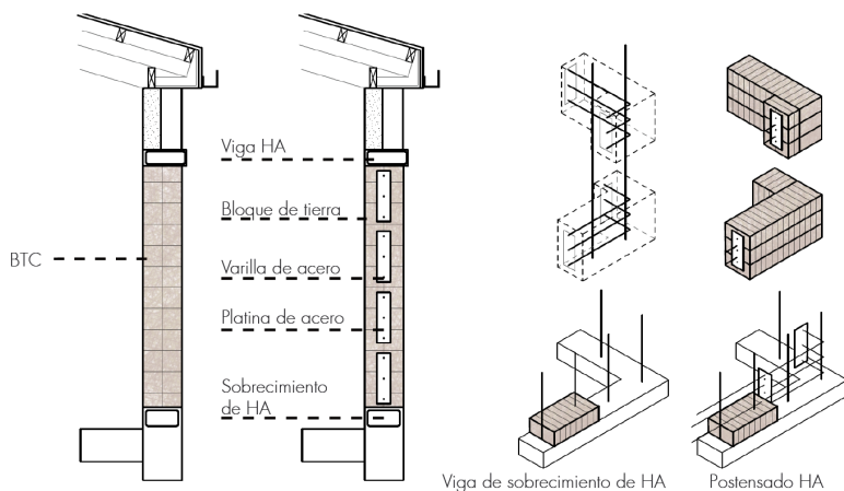
Fig. 2.5.5 | El uso de los bloques en sinergia con elementos estructurales de acero y hormigón. | Fuente: Autoría Propia (2024).
