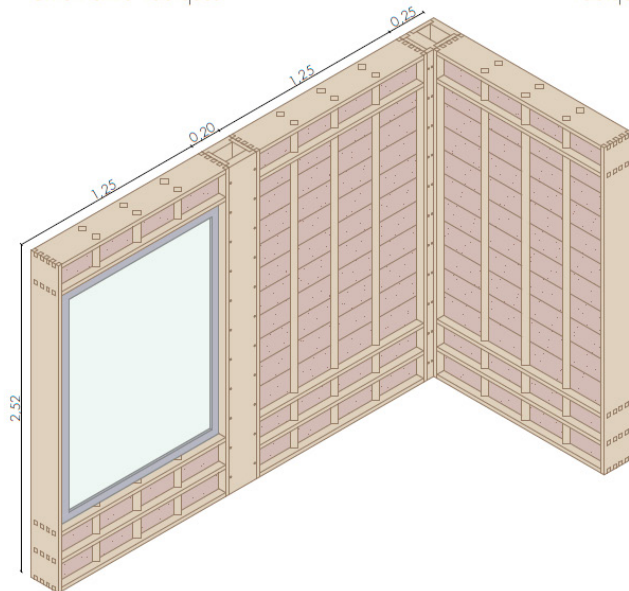
Unión entre tabiques en encuentro en esquina y tabique con ventana
