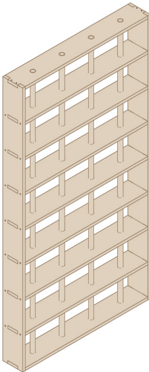
Armazón para muro de bloques
