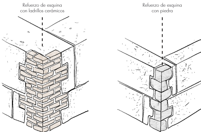
Fig. 2.2.17 | Fortalecimiento de esquinas con mampuestos más resistentes. | Fuente: AutoríaPropia.(2024).
