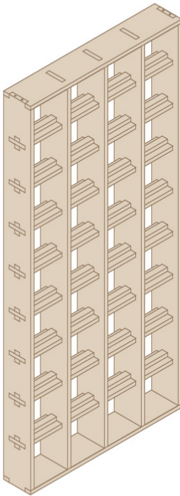
Armazón para muro de bloques
