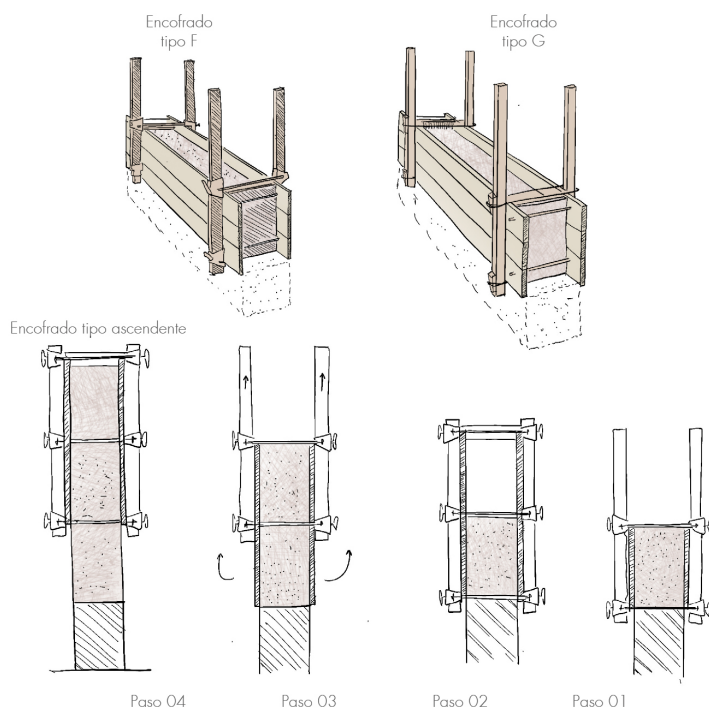
Fig. 2.4.9 | Ejemplos de diferentes sistemas de encofrados. | Fuente: Autoría Propia (2024).
