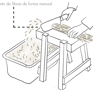
Corte de fibras con guillotina
