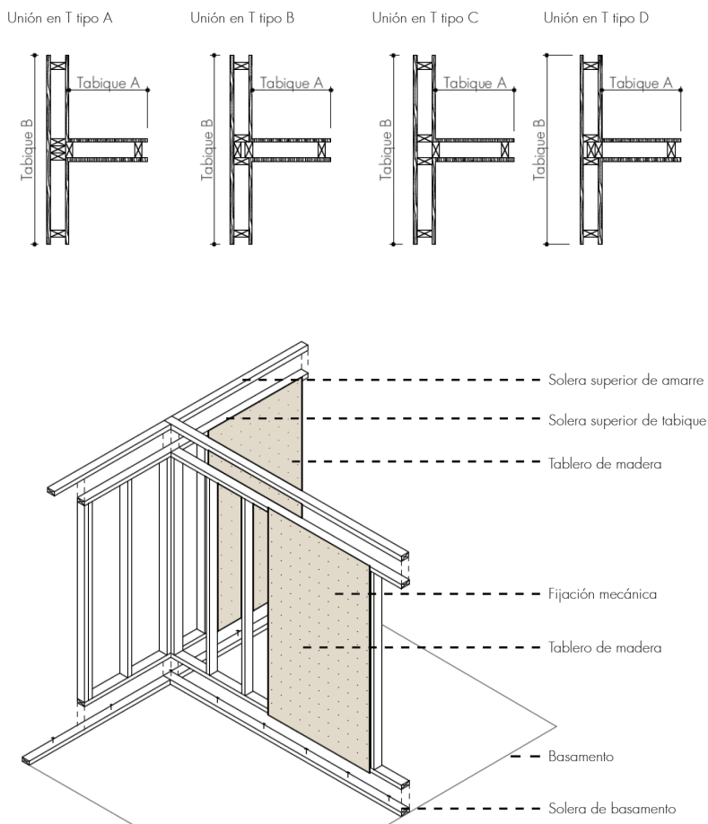
Fig. 3.3.10 | Diferentes tipos de uniones entre tabiques con bastidores B. | Fuente: Autoría Propia (2024).
