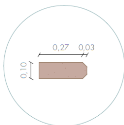
BLOQUE TIPO 1 Material: Tierra Comprimida Cantidad: 32 unidades
