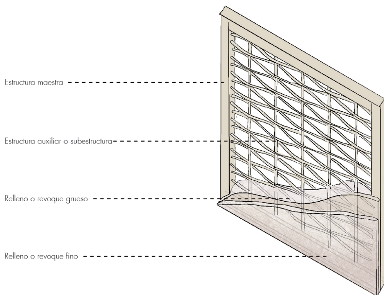
Fig. 2.3.9 | Partes que conforman un tabique con entramados y barro | Fuente: Autoría Propia (2024).
