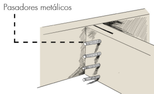
Fig.3.3.11 | Unión con pasadores. | Fuente: Autoría Propia (2024).
