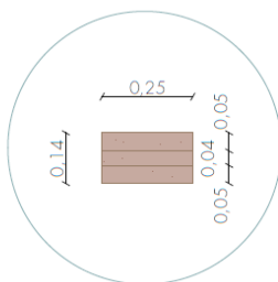
BLOQUE TIPO 2 Material: Tierra Comprimida Cantidad: 8 unidades
