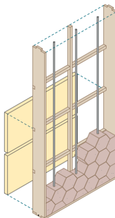
Paso 2 Instalación de bloques y aislante.
