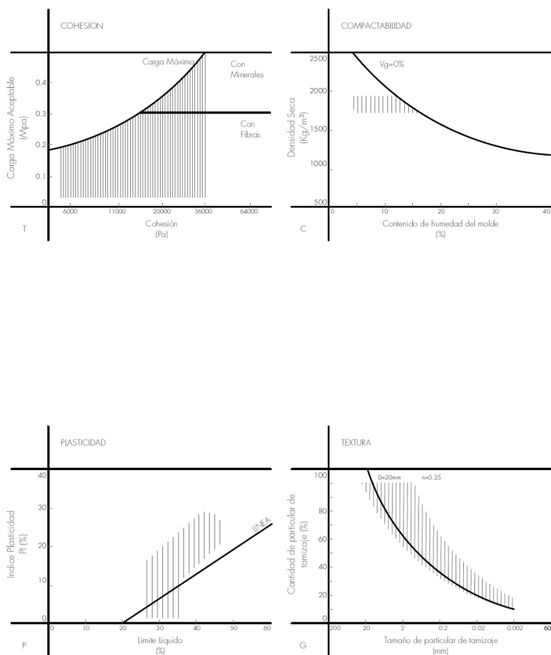
Fig. 2.4.5 | Características del suelo recomendado para tierra apisonada. | Fuente: Houben y Guillaud, (2008).
