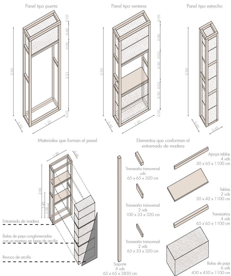
Fig.2.5.8 | Tabique con elementos compuestos con paja y revocos de arcilla. | Fuente:Autoría Propia(2024)
