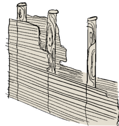
b) Panel hueco con tejido de latillas horizontales listas para revoque.
