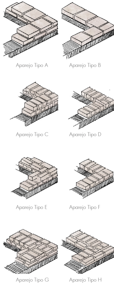
Fig. 2.2.14 | En la configuración de tabiques es importante el trabajo de aparejo de adobes. | Fuente: Autoría Propia. (2024).
