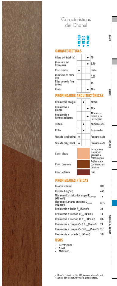
Fig. 3.3.25 | Características del chanul. | Fuente: Arpi, et al. (2018).
