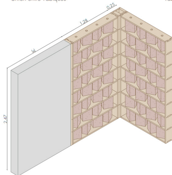
Unión entre tabiques en encuentro en esquina y tabique con ventana
