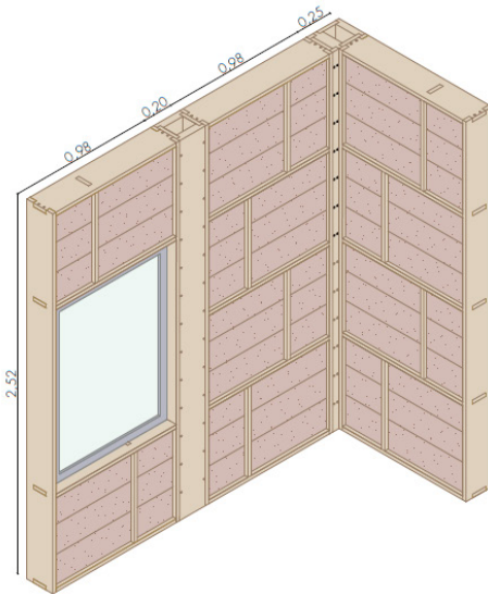
Unión entre tabiques en encuentro en esquina y tabique con ventana
