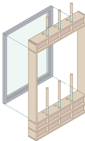
Paso 4 Listones frontales y ventana dentro de la estructura del tabique.
