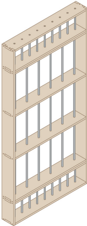
Armazón para muro de bloques
