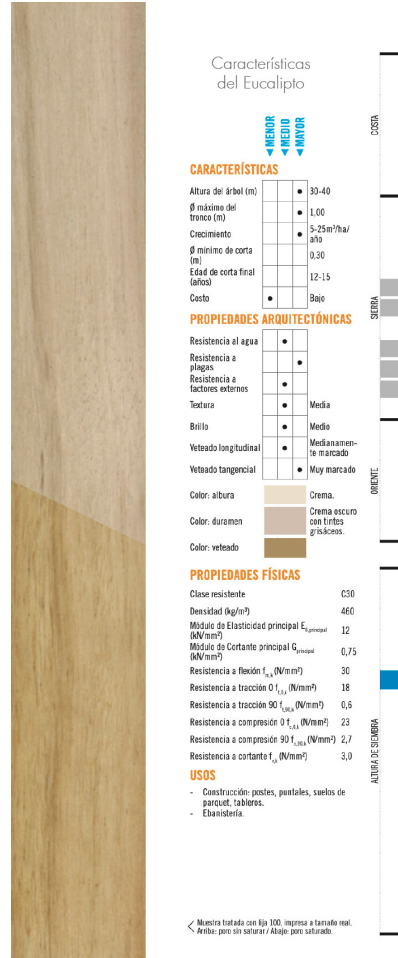
Fig. 3.3.26 | Características del eucalipto. | Fuente: Arpi, et al. (2018).
