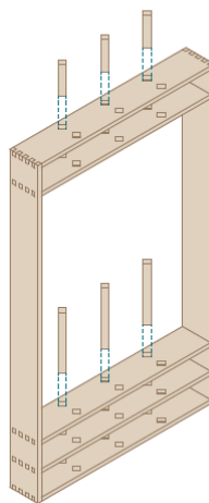
Paso 2 Listones posteriores.
