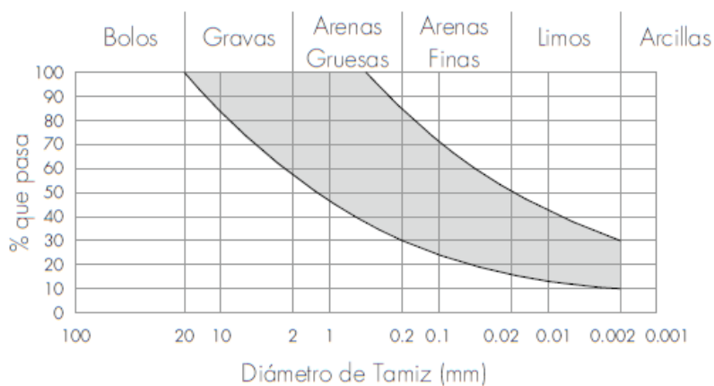
Fig.3.2.13 | Granulometría recomendada de tierras para fabricación de BTC. | Fuente: Minke, (2006).
