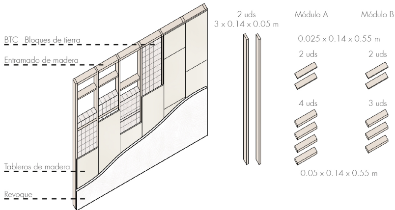
Fig. 2.5.6 | Tabi ques con BTC empleados por la oficina de arquitectura Schauer+Volhard en Alemania. | Fuente: Autoría Propia (2024).
