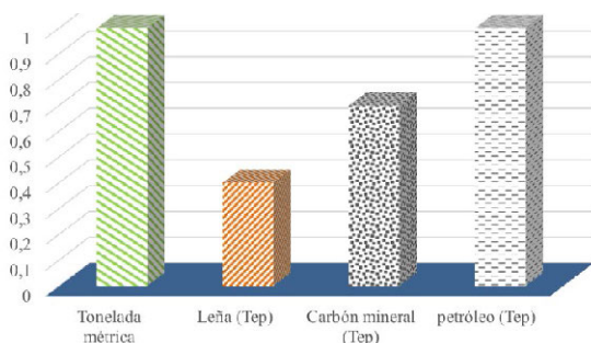
Figura 2. Densidad energética relativa de los portadores primarios
