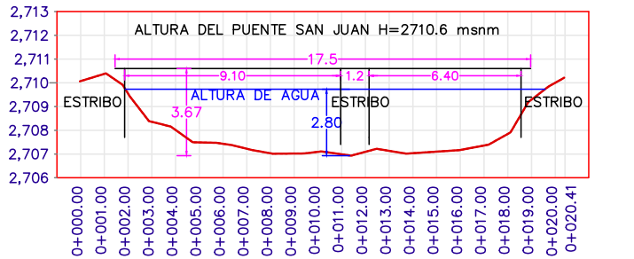
Figura 11.1. Secciones transversales del puente San Juan 3+200
