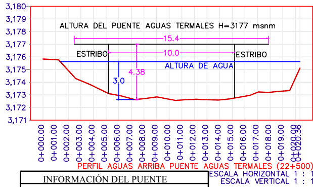
Figura 25.1. Secciones transversales del puente Aguas Termales 22+500
