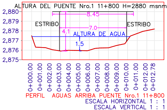
Figura 17.1. Secciones transversales del puente N° 1 11+800
