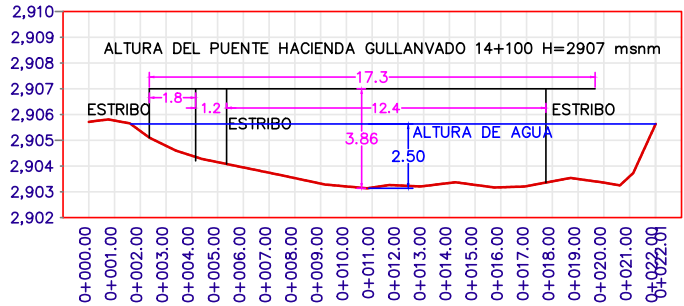
Figura 20.1. Secciones transversales del puente Hacienda Gullanvado 14+100
