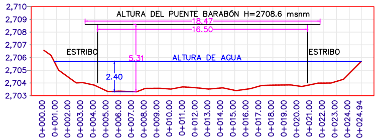
Figura 10.1. Secciones transversales del puente Barabón 3+000
