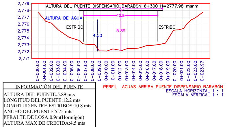
Figura 14.1. Secciones transversales del puente Dispensario Barabón 6+300
