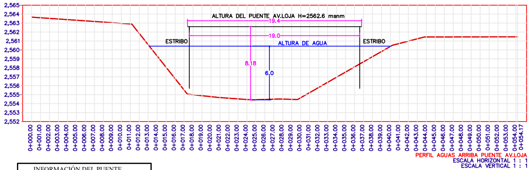
Figura 5.1. Secciones transversales del puente Av. Loja
